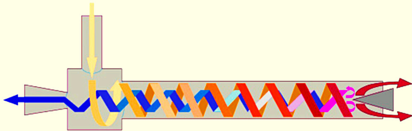
Рис. 2.1 Схема поділу потоків повітря у вихровій трубі [5; 10]
